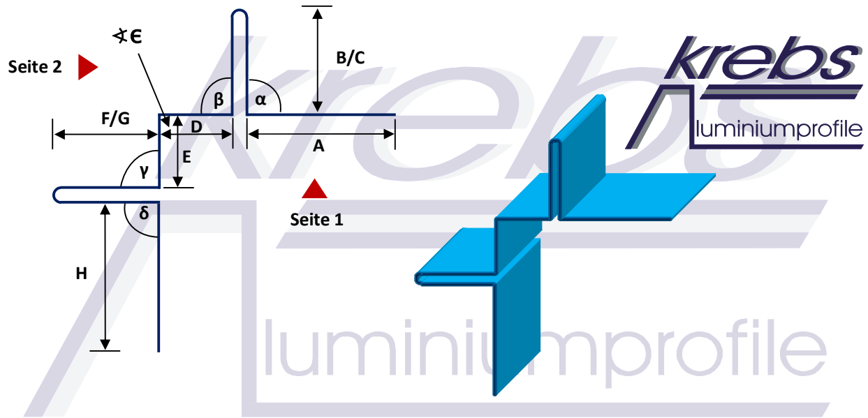
Abkanteilmaße
